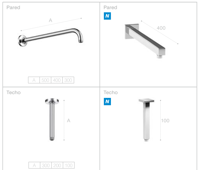
Brazo soporte a pared/techo no incluido en rociadores. Medidas en mm.
